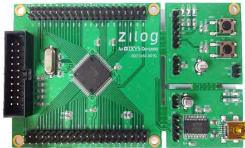
Figure 2. Mini Board
